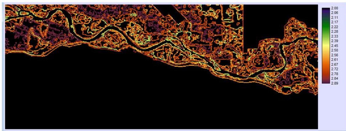
Figura N° 7. Dimensión fractal
